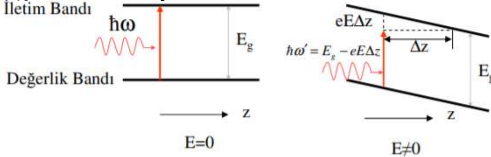
Franz-Keldysh Etkisi
